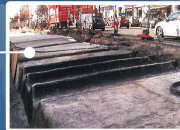
Tunnelabdichtung, Berlin U2 - Kaiserdamm
